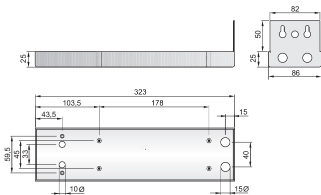
Konsole K 143-S/Bracket K 143-S
