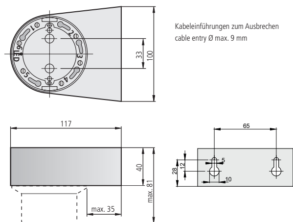
Konsole K 143-K/Bracket K 143-K
