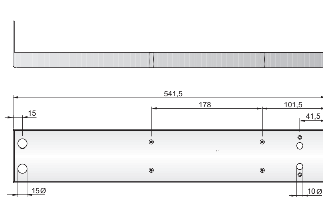
Konsole K 143-K/Bracket K 143-K
